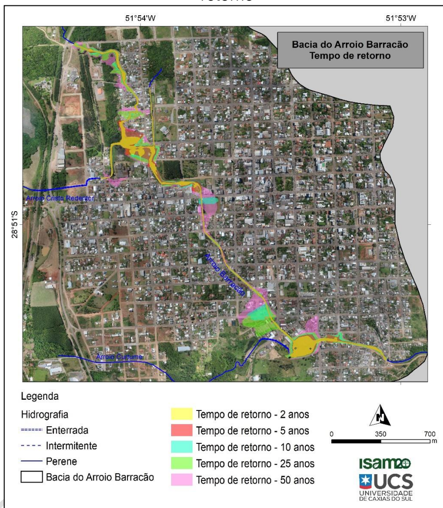
Figura 92 – Resultado das manchas de inundação para diferentes períodos de retorno
