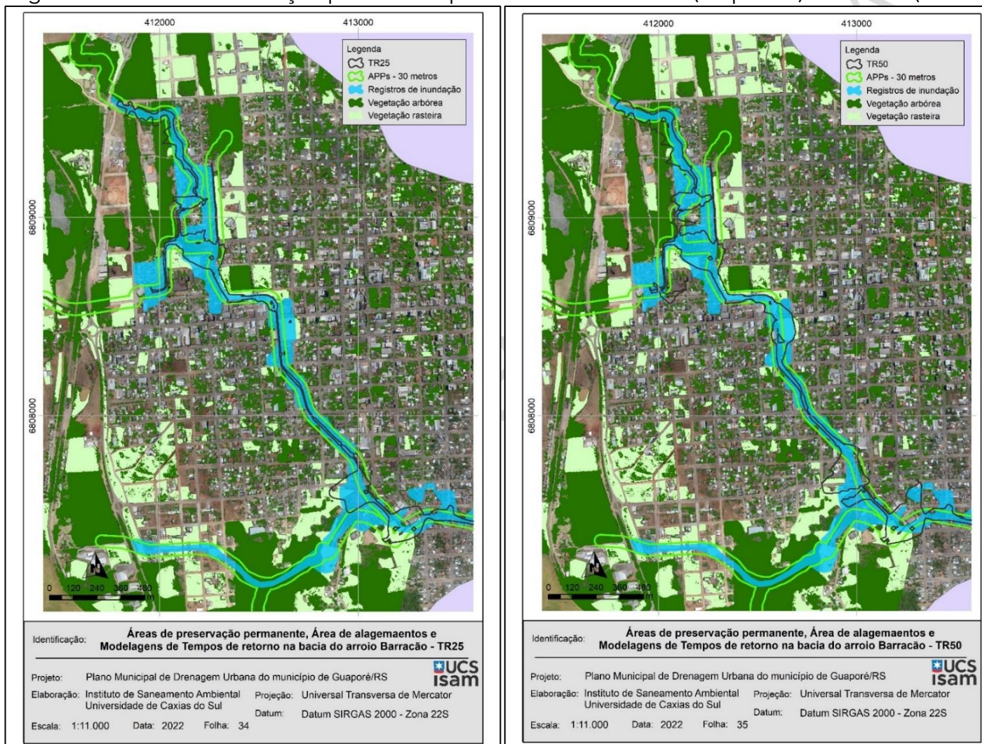
Figura 98 – Área de inundação para os tempos de retorno 25 anos (esquerda) e 50 anos (direita)
