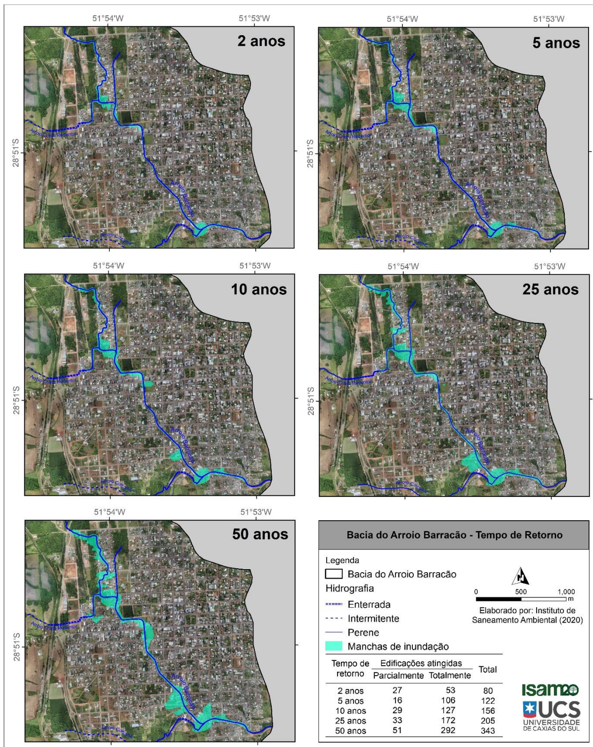
Figura 93 – Resultado das manchas de inundação para diferentes períodos de retorno
