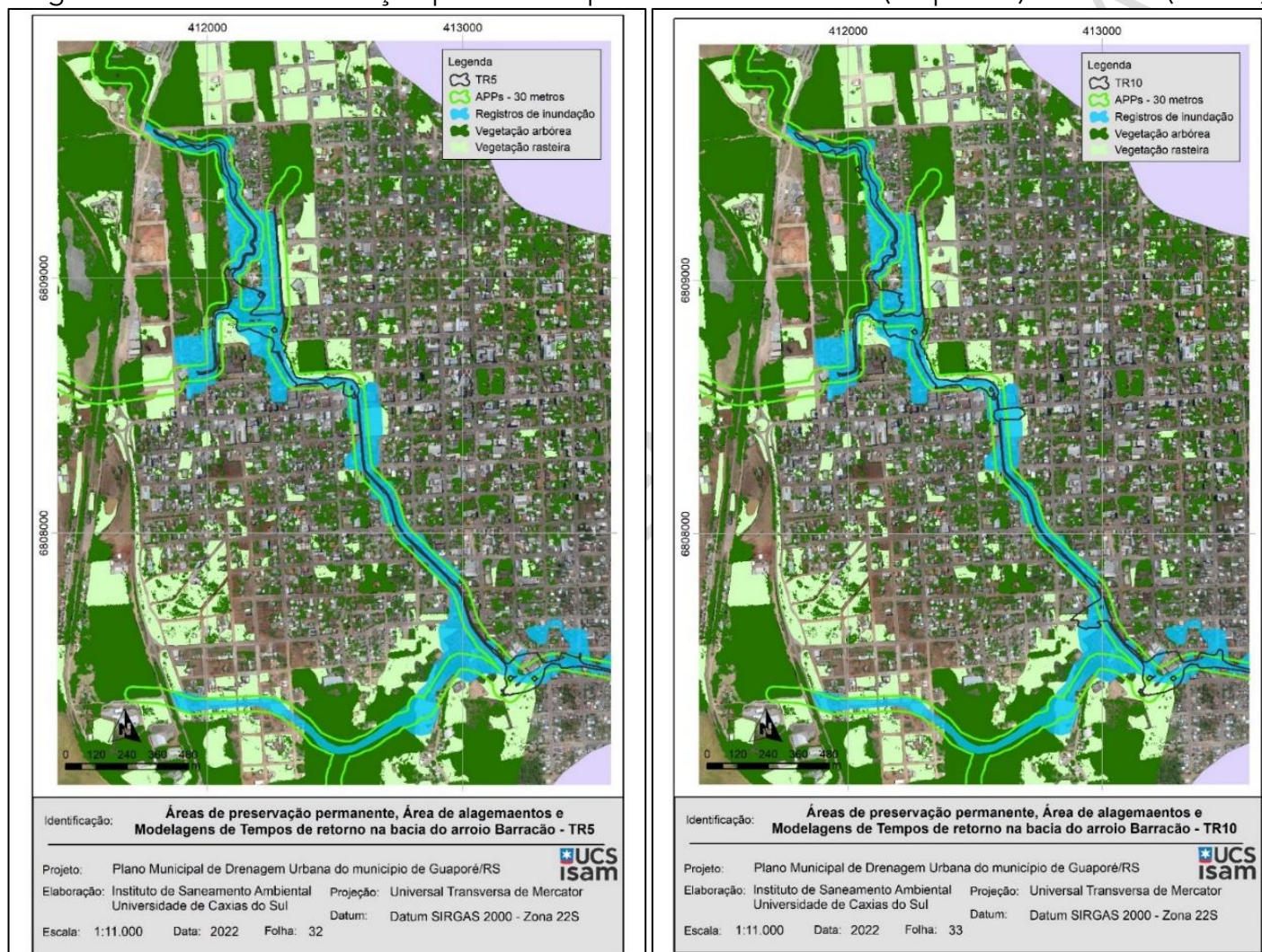
Figura 97 - Área de inundação para os tempos de retorno 5 anos (esquerda) e 10 anos (direita)
