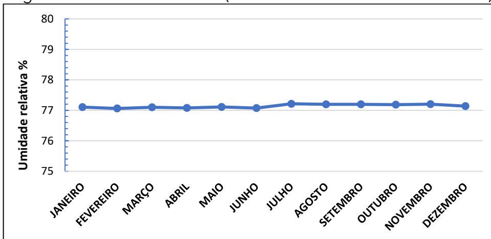
Figura 66 - Umidade relativa (média mensal dos últimos 30 anos)
