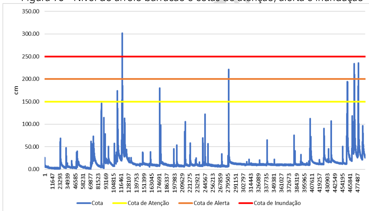
Figura 95 – Nível do arroio barracão e cotas de atenção, alerta e inundação
