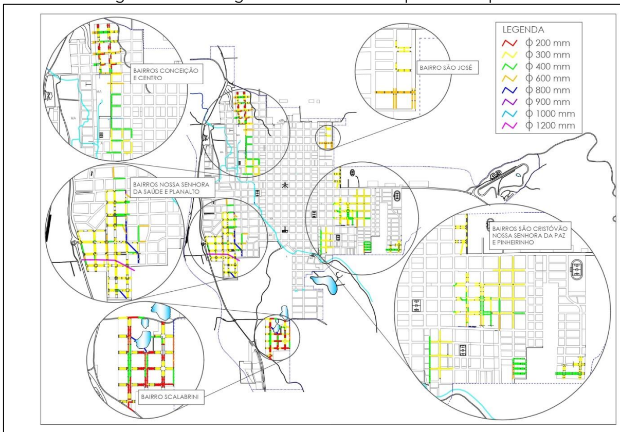
Figura 79 – Drenagem urbana do município de Guaporé
