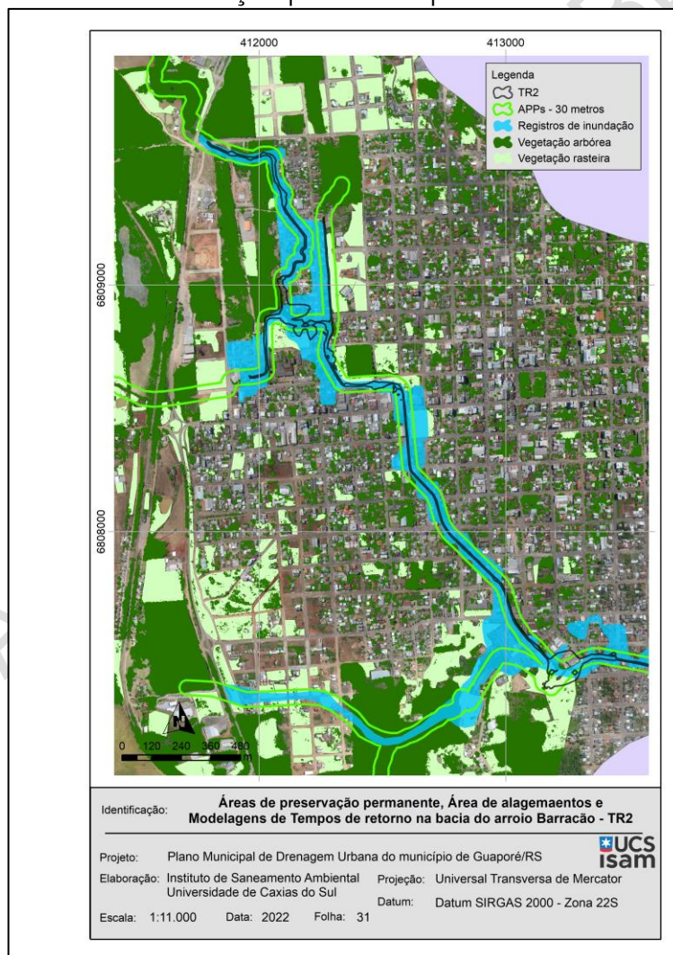
Figura 96 - Área de inundação para o tempo de retorno 2 anos
